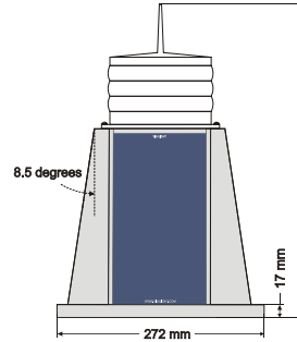
Đèn mạn trái (Port side)
